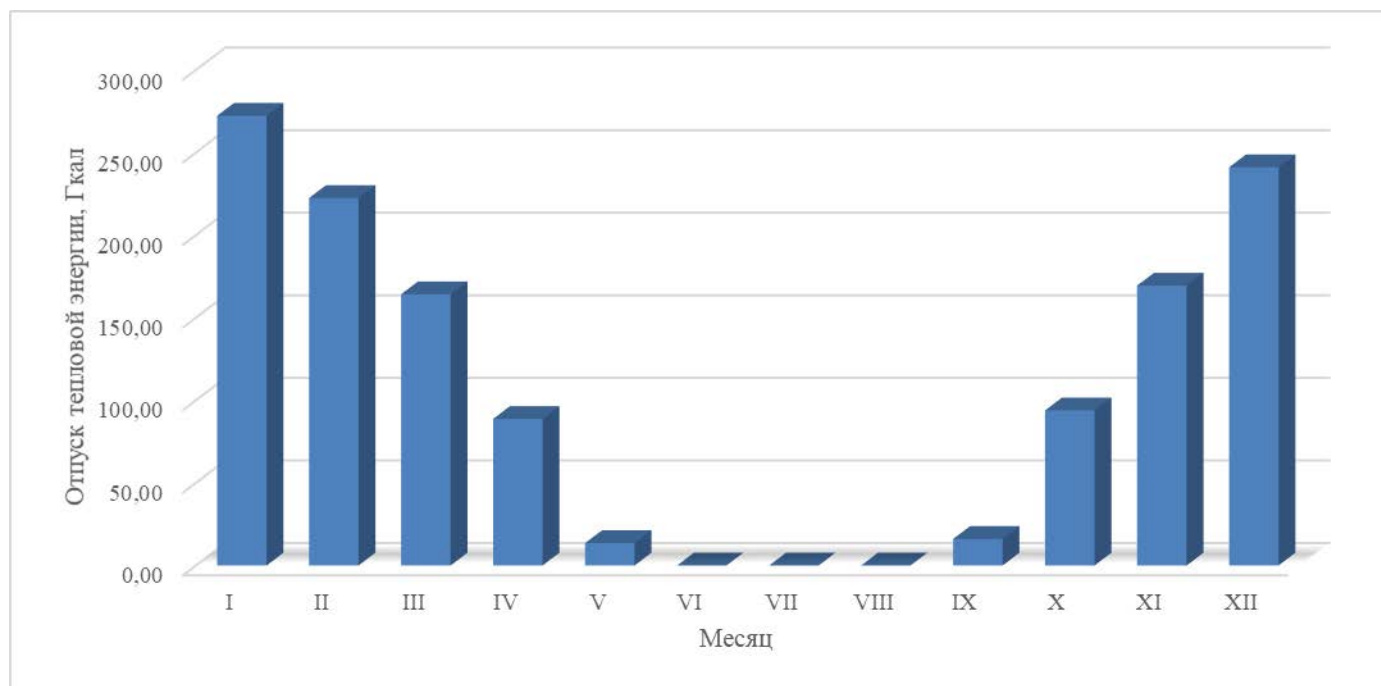
Рисунок 1.2 – Оптимальный температурный график отпуски тепловой энергии по котельной с. Ягодное
