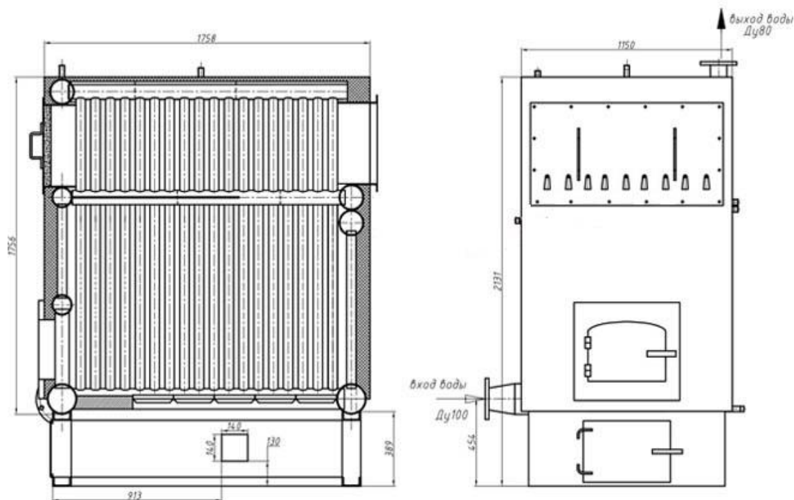
Рисунок 2.1 – Котел КВР 0,5 КБ
