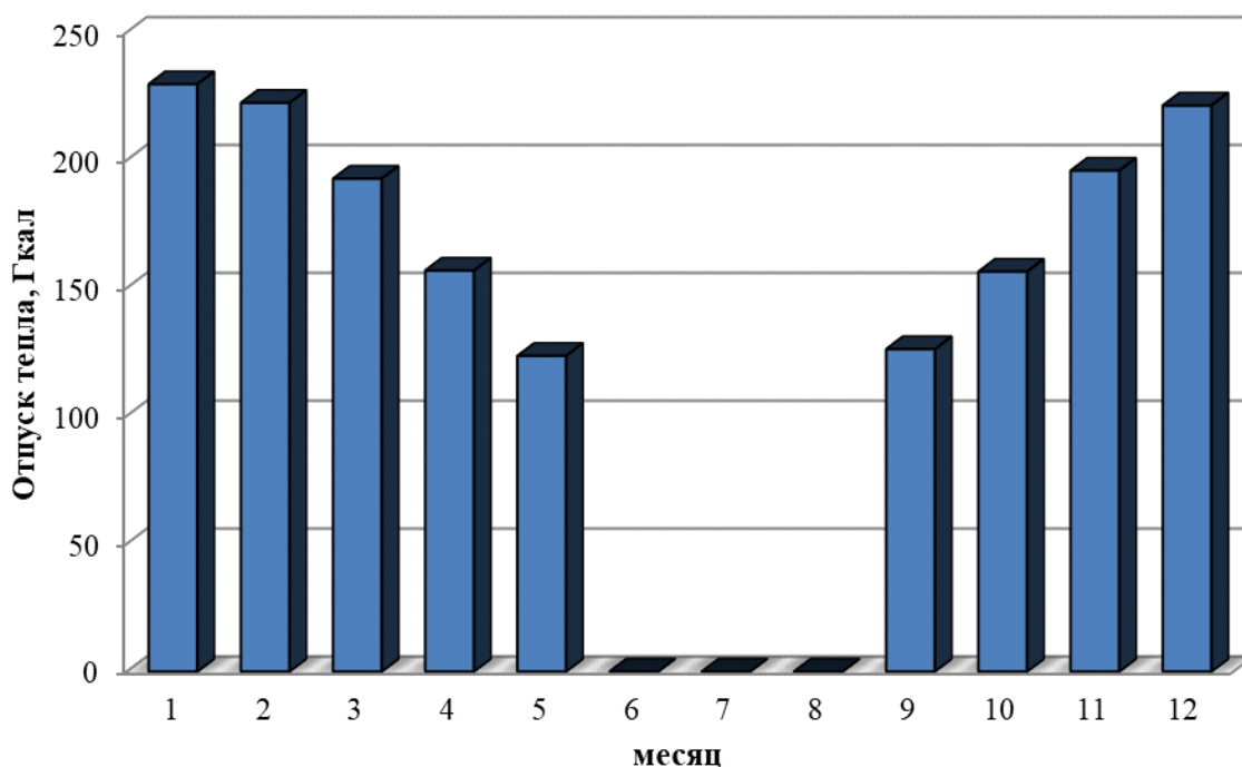
Рисунок 1.2 – Оптимальный температурный график отпуски тепловой энергии для поселковой котельной Ягодного сельского поселения
