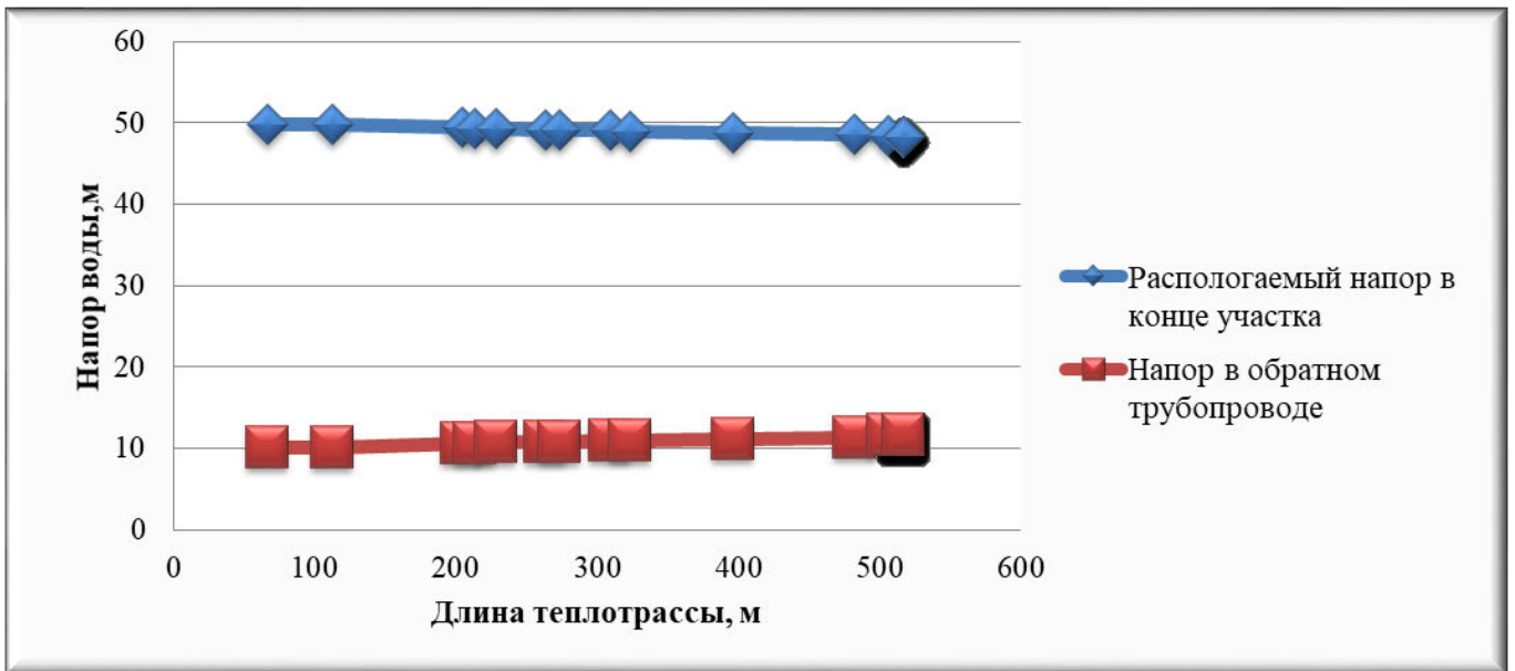
Рисунок 2.5 – Пьезометрический график тепловой сети поселковой котельной с. Ягодное по магистральному выводу
