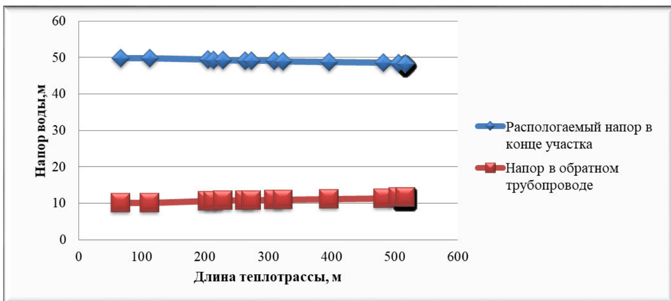
Рисунок 2.4 – Пьезометрический график тепловой сети поселковой котельной с. Ягодное по магистральному выводу
